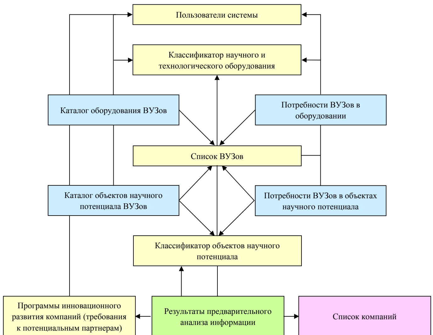
Рис. 1. Структурно-функциональная схема электронного каталога
